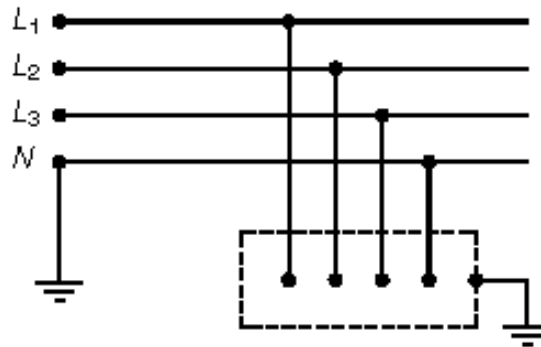
Sistema TT
