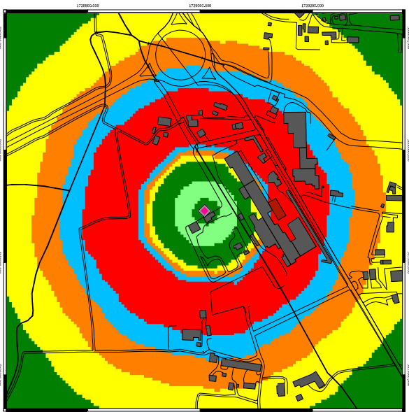
Campo elettromagnetico (V/m) calcolato alla quota di 12,3 m sul livello del terreno
