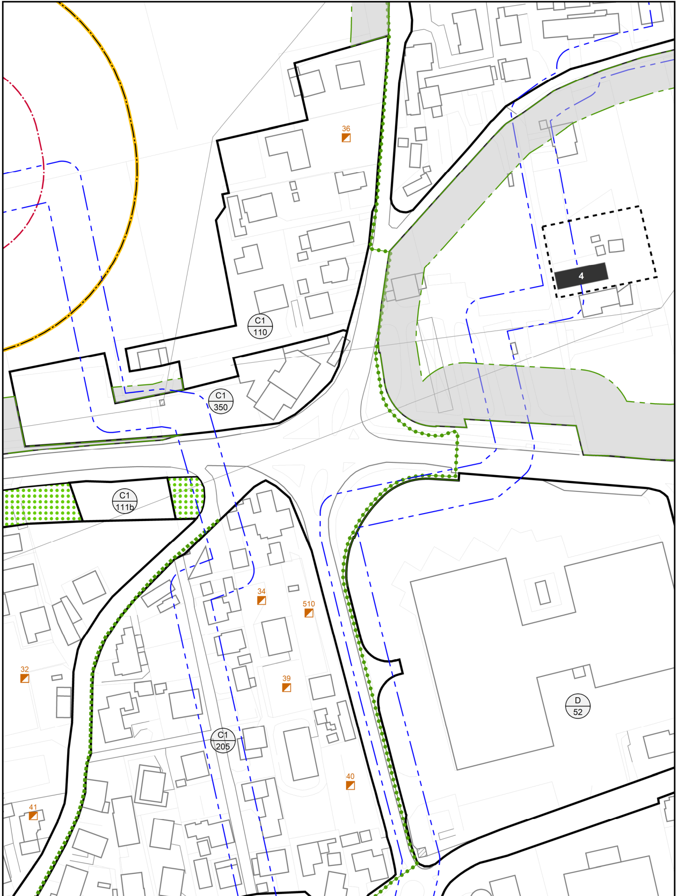
OP 1210 REALIZZAZIONE ROTATORIA TRA SR 53 E VIA DEL COMMERCIO Stato di variante
