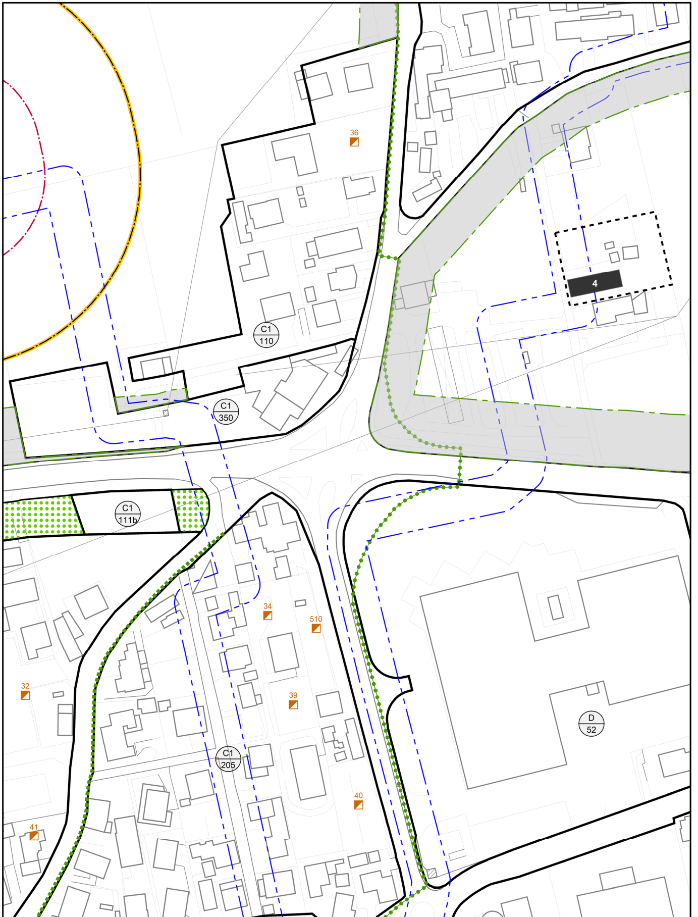
OP 1210 REALIZZAZIONE ROTATORIA TRA SR 53 E VIA DEL COMMERCIO Stato attuale
